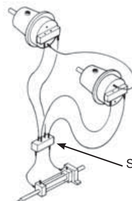
In-bord avec soupape MRD4 (dans le cas d'une pompe sans soupape de blocage)
