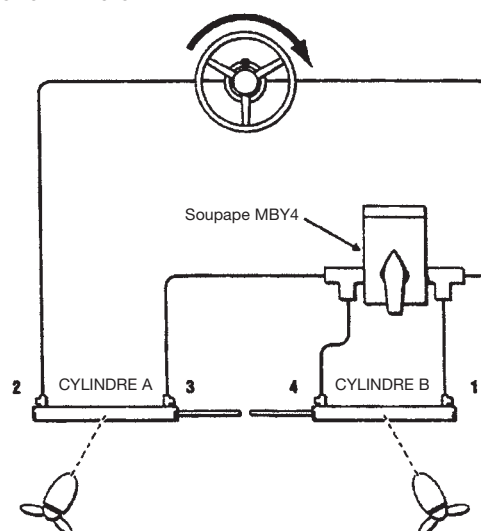
CYLINDRES NON-BALACÉS
