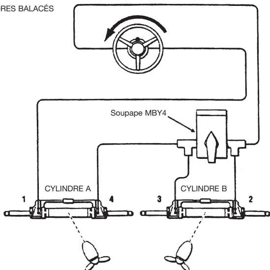
CYLINDRES BALACÉS
