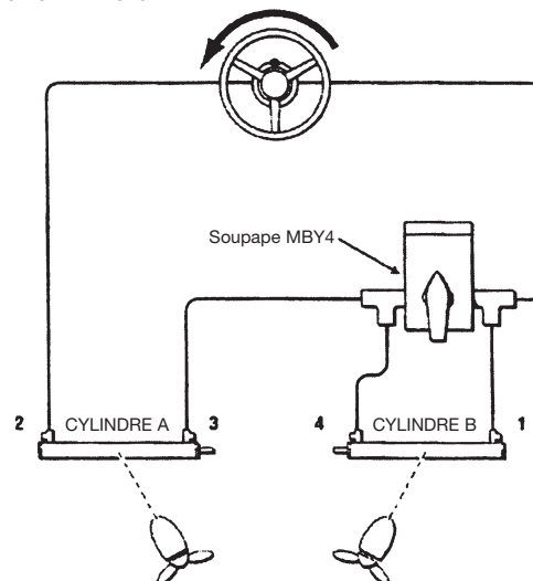
CYLINDRES NON-BALACÉS
