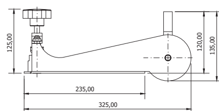
Musone in acciaio inox AISI 316 lucidati a specchio lungh. 330 largh. 80 sp. 4 mm con 1 bloccaggio. Per ancore Bruce/ Danforth fino a 10 Kg Cod. 229.06 Polished stainless steel AISI 316 bow roller length 330 width 80 thickness 4 mm with bloking device. For anchors Bruce/ Danforth up to 10 Kg Cod. 229.06
