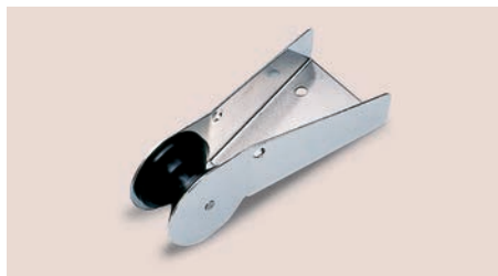
Musone di prua inox modello piccolo. Per ancore fino a 7,5 Kg S.s. bow roller small model. For anchors up to 7,5 Kg
