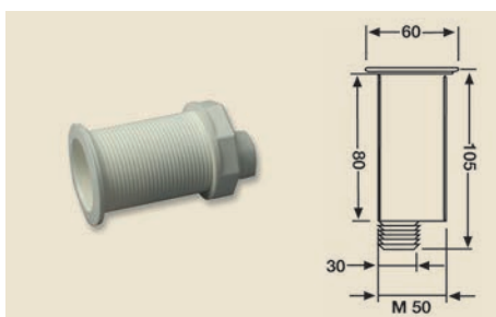
Boccola di scarico fabbricata in nylon bianco. Plastic through deck fitting
