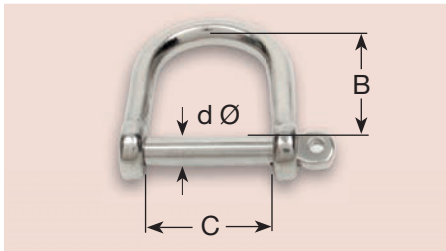
Grilli acc. inox tipo largo.
