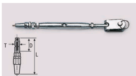
Tenditori acc. inox con terminale rapido. Rigging screws with swageless stud terminal.
