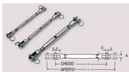
Tenditori acc. inox con canaula chiusa. Rigging screws closed body toggle.
