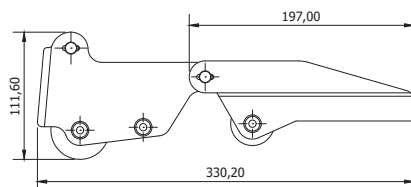
Musone inox Stainless steel anchor roller Per ancore fino a 10 Kg For anchors up to 10 Kg
