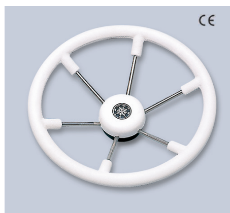
Cod. V.AB34 Ø 330 dis F Cod. V.AB36 Ø 360 dis L Cod. V.AB40 Ø 400 dis L Volante a 6 razze con impugnatura in poliuretano colore bianco.
